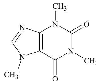
3. Caffeine
